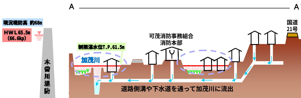
図- 2.1.4 下流域の地形的特徴（断面横断模式図）
