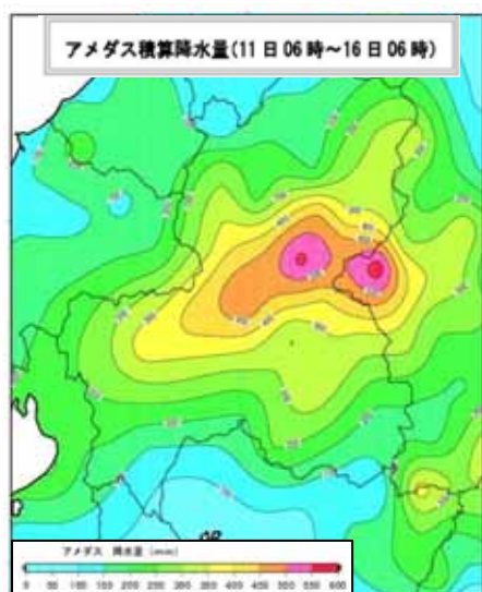
付図-2 平成 22 年 7.15 豪雨概況
